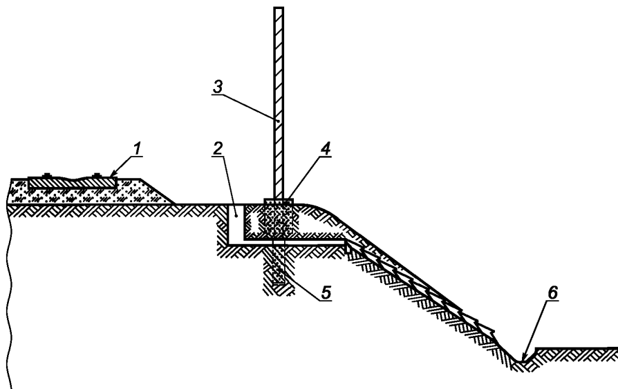
1 — железнодорожный путь; 2 — водооток; 3 — акустический экран; 4 — бетонное основание; 5 — свая для закрепления фундамента акустического экрана; 6 — лоток для отвода воды
